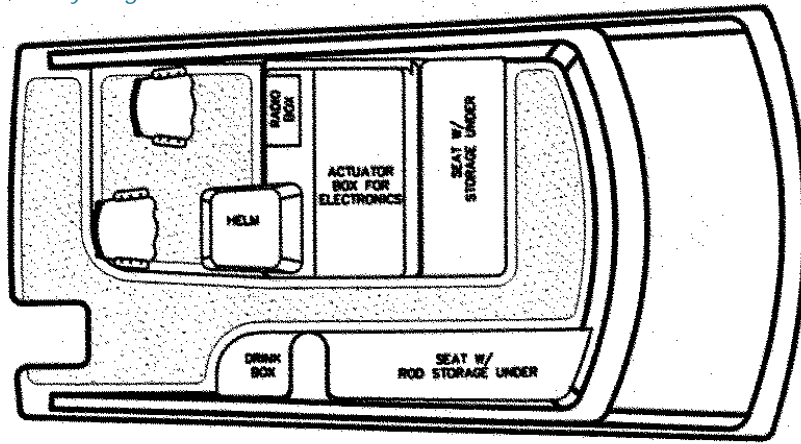
Flybridge Plan ▼
